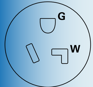
265 VOLT PLUG 277 VOLT CONFIGURATION 5.0 KW HEATER – 30 AMP BREAKER NEMA 7-30
