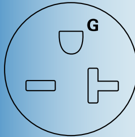
230/208 VOLT PLUG 250 VOLT CONFIGURATION 3.4 KW HEATER – 20 AMP BREAKER NEMA 6-20 T-SLOT (2)
