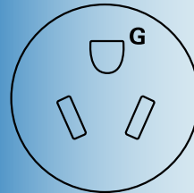
265 VOLT PLUG 277 VOLT CONFIGURATION 3.4 KW HEATER – 20 AMP BREAKER NEMA 7-20
