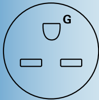
230/208 VOLT PLUG 250 VOLT CONFIGURATION 2.5 KW HEATER – 15 AMP BREAKER NEMA 6-15
