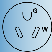
265 VOLT PLUG 277 VOLT CONFIGURATION 2.3 KW HEATER – 15 AMP BREAKER NEMA 7-15
