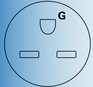
230/208 VOLT PLUG 250 VOLT CONFIGURATION 5 KW HEATER – 30 AMP BREAKER NEMA 6-30
